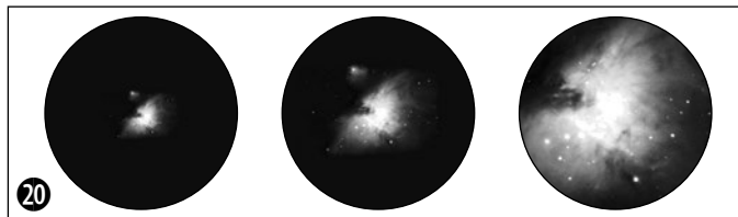
Orion-Nebel (M 42)
